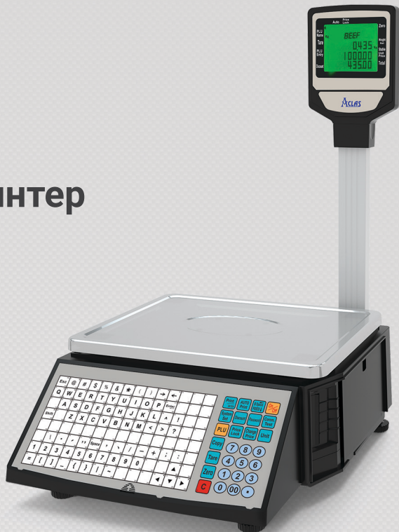
Етикетираща везна с изнесени дисплеи LS2ZC
